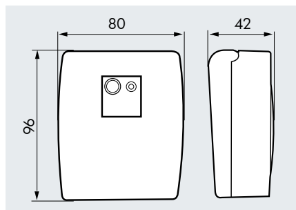
Socle pour le montage sur mât (inclus)
