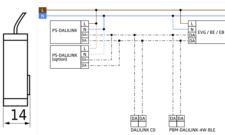
Schéma de raccordement
